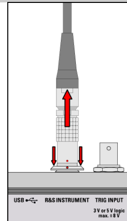
Bild 1-6 Entriegeln des R&S Instrument-Anschlusses
